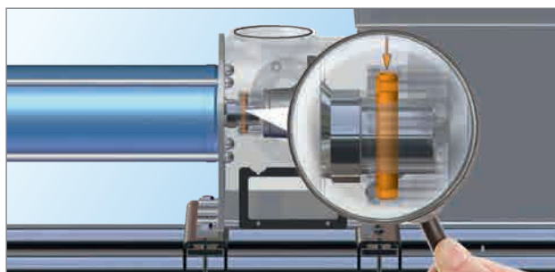
Étape 1 : Desserrer les vis de fermeture et retirer les boulons de raccordement.
