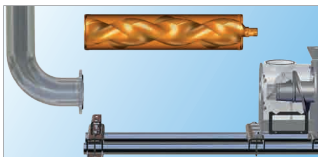
Étape 3 : Déplacer le stator et le rotor vers l'avant et sortir du carter de la pompe.
