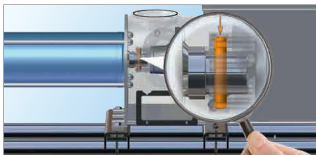
Krok 1: Odkręcić śrubę maskującą i usunąć bolec łączący przegub Cardana z wałem.
