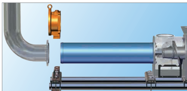
Krok 2: Poluzować pręty ściągające po stronie tłocznej, wyciągnąć kołnierz wylotowy do góry.
