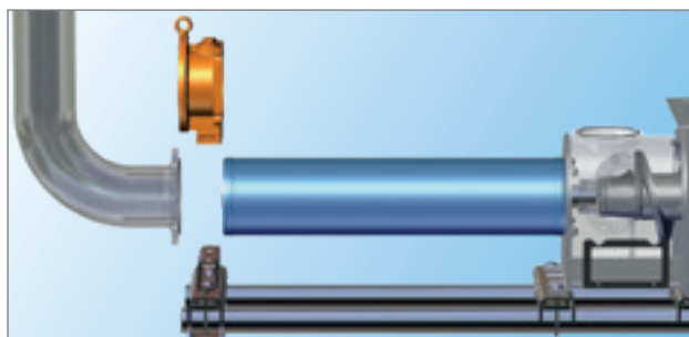
Шаг 2: Открутите крепеж нагнетательного патрубка, снимите его, подняв его вверх
