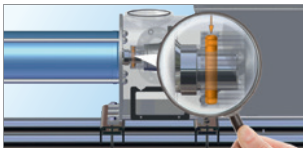
Шаг 1: Выбейте шпонку, фиксирующую карданный и приводной валы.
